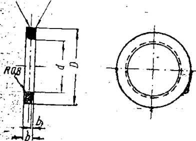
Шайба уплотнительная
