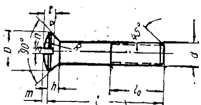
Винт для металла с полупотайной головкой
