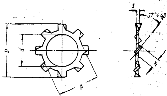
Шайба пружинная плоская с наружными зубцами
