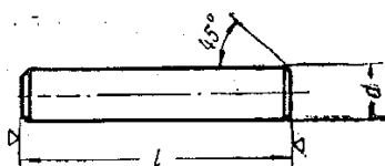
Штифт
