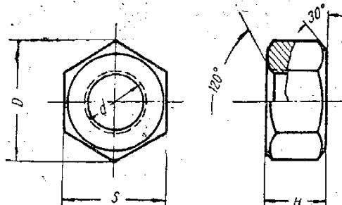
Гайка
