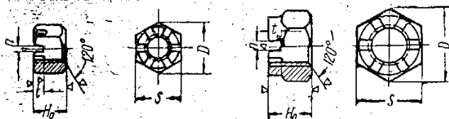
Гайка корончатая
