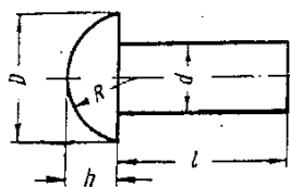
Заклепка с полукруглой головкой
