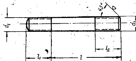
Шпилька
