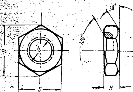
Гайка низкая
