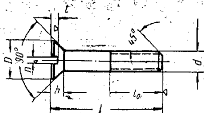
Винты для металла с потайной головкой
