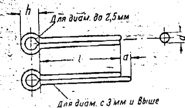
Шплинт разводной
